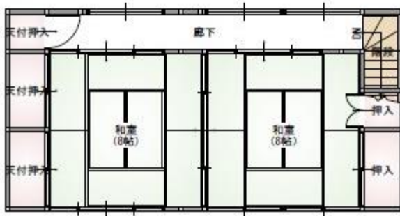
2階 平面図 S:1/100
